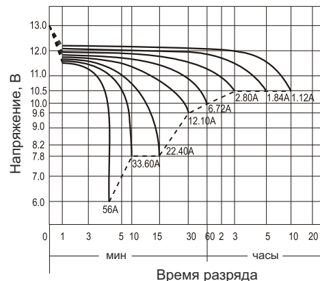
Разрядные характеристики
